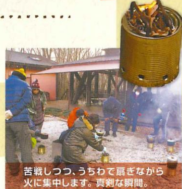
ウッドガスストーブを実際に使っておいしいご飯が炊けました!!
